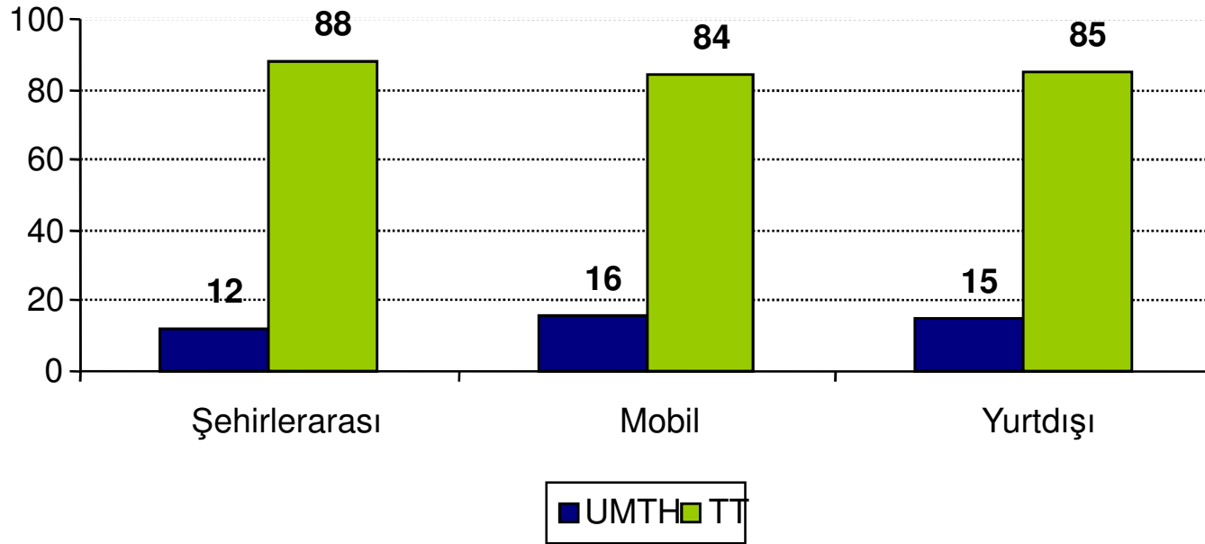
UMTH-TT Çağrı Başlatma Trafik Kiyaslaması, 2008-2
